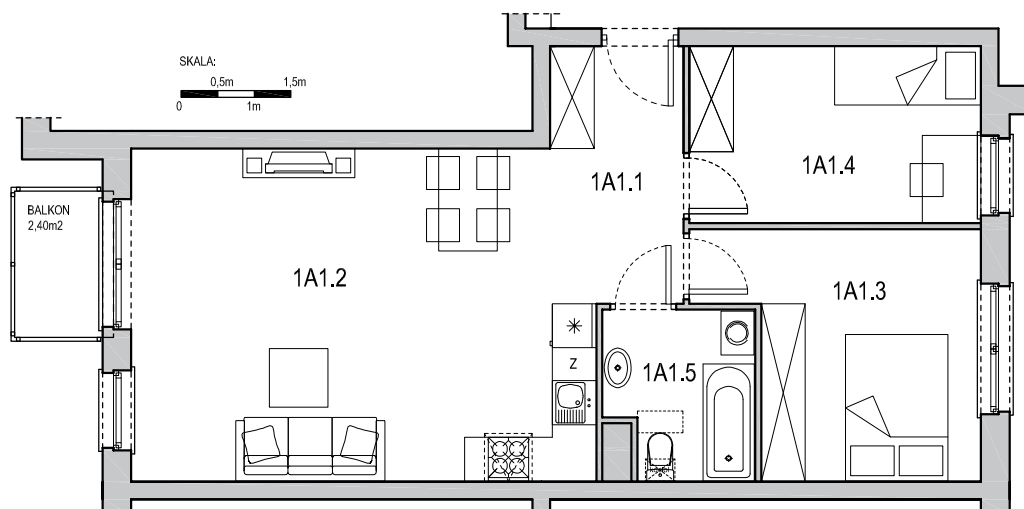
RZUT MIESZKANIA
