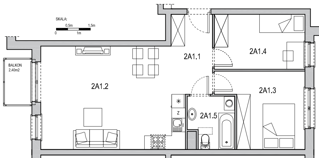
RZUT MIESZKANIA
