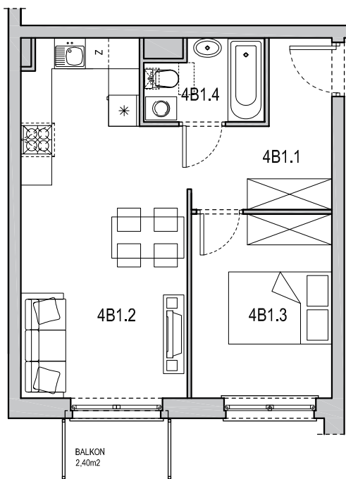
RZUT KONDYGNACJI -LOKALIZACJA MIESZKANIA
