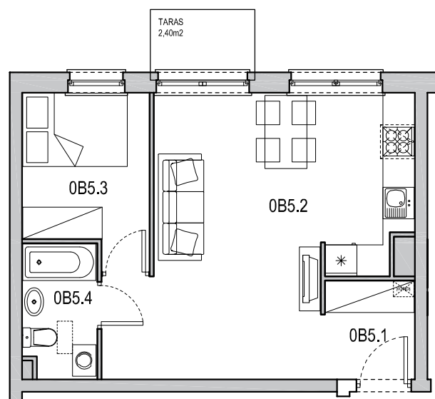
RZUT MIESZKANIA
