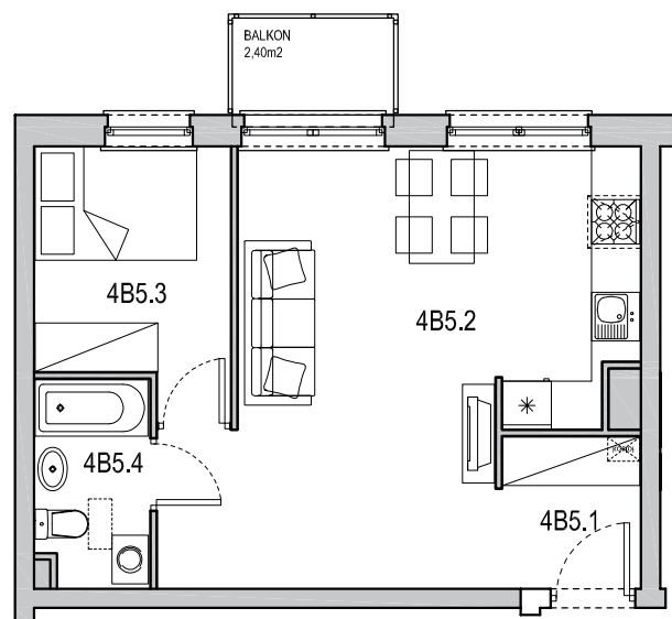
RZUT MIESZKANIA
