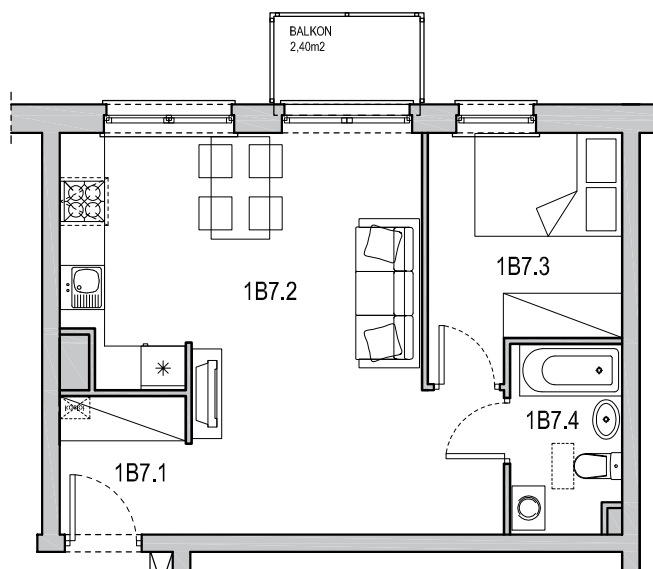
RZUT MIESZKANIA
